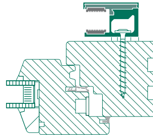
Befestigungsvariante bei Holzfenstern
