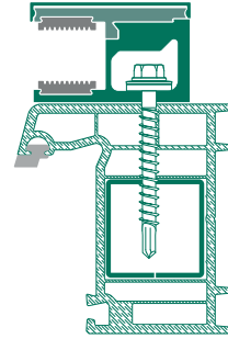
Befestigungsvariante bei Kunststofffensterprofilen
