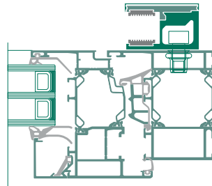
Befestigungsvariante bei Aluminiumfenster
